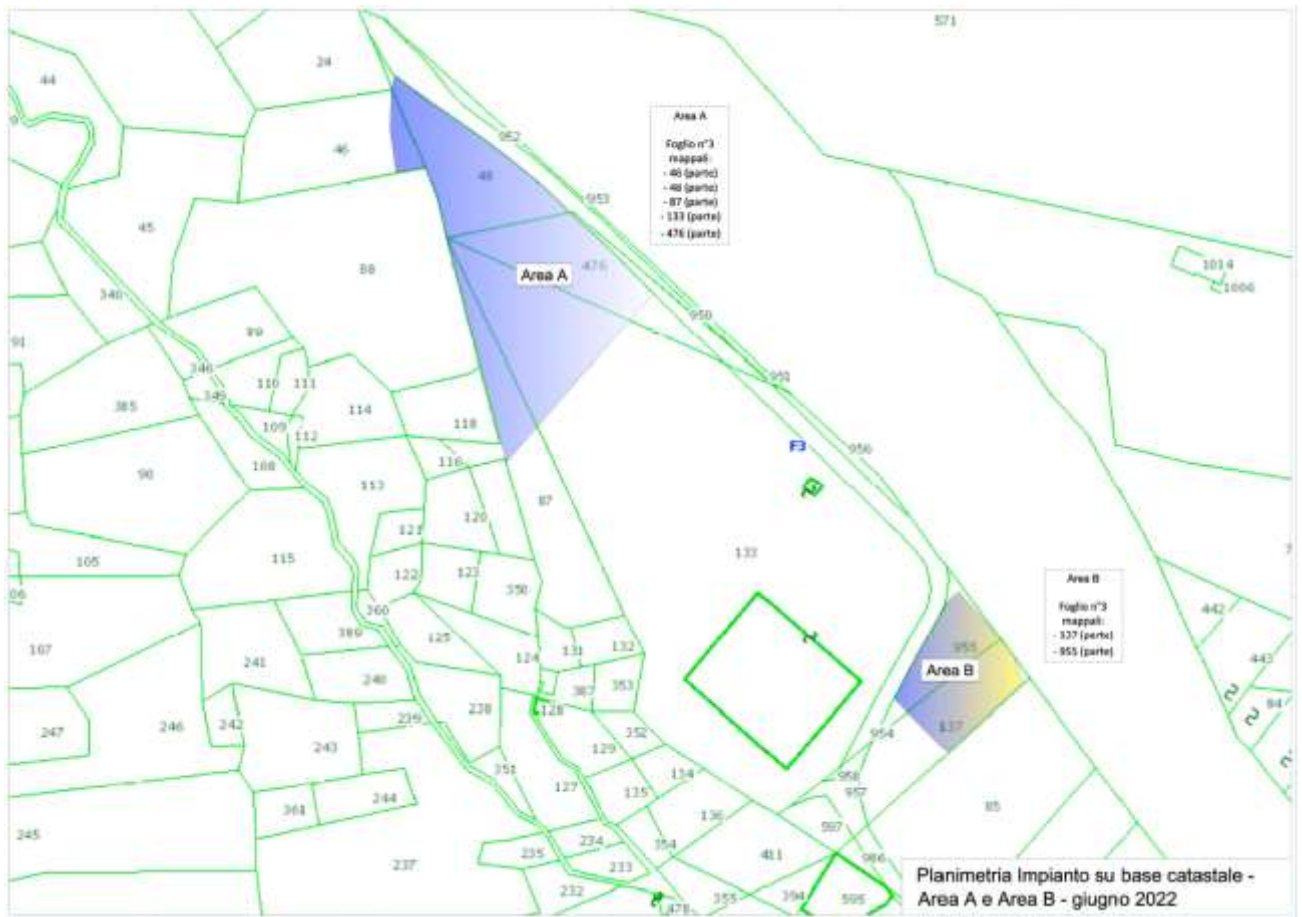
Figura 2 Planimetria impianto su base catastale Ortofoto area di interesse
